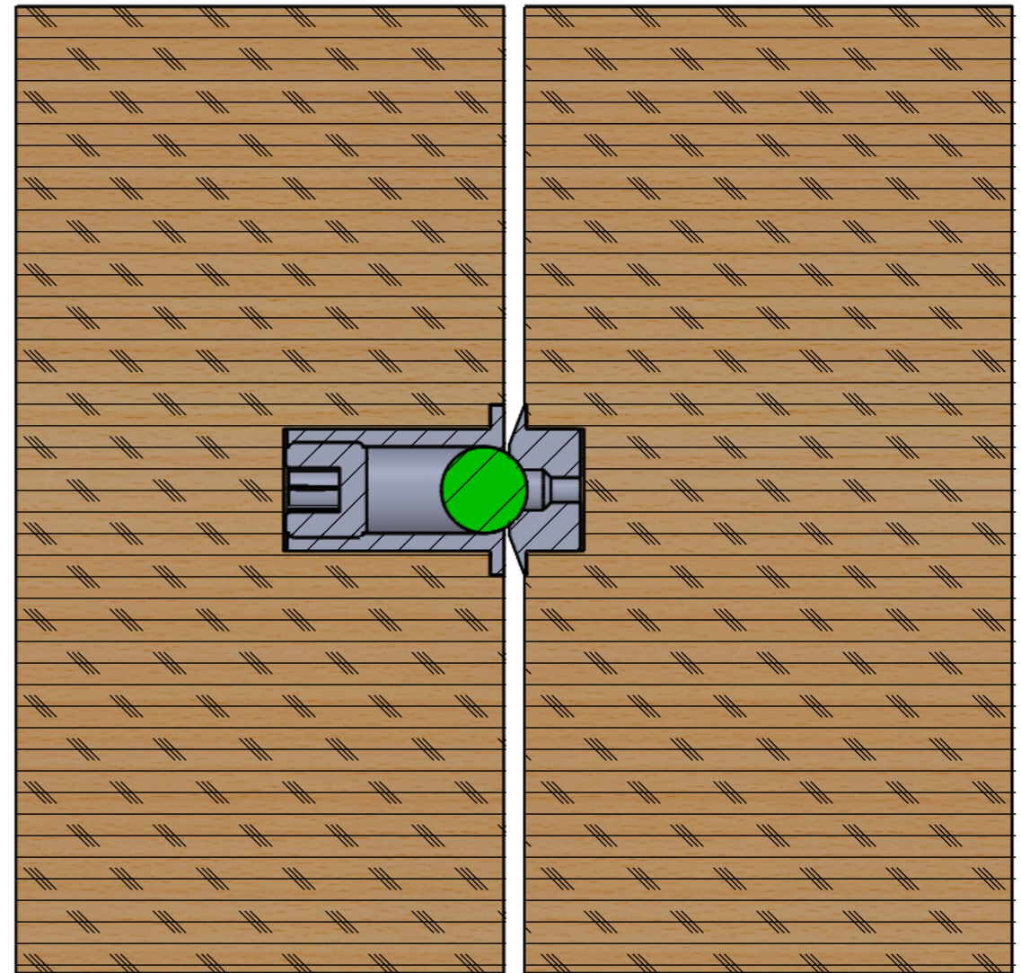
SEZIONE A-A SCALA 1:1
